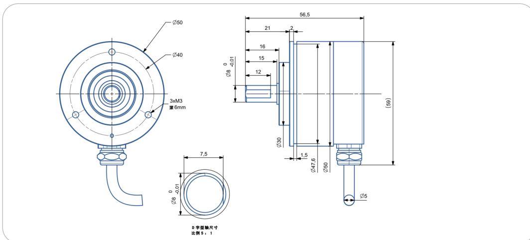
尺寸型号图7：输出轴8mm IP68/防爆
