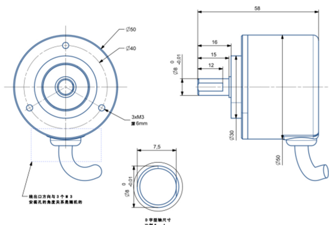
尺寸型号图4：输出轴8mm IP54
