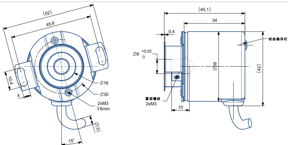
尺寸型号图2：输出轴8mm盲孔IP54
