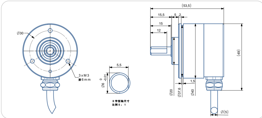
尺寸型号图5：输出轴6mm IP68/防爆
