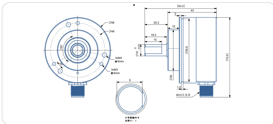
尺寸型号图9：输出轴10mm IP68/防爆
