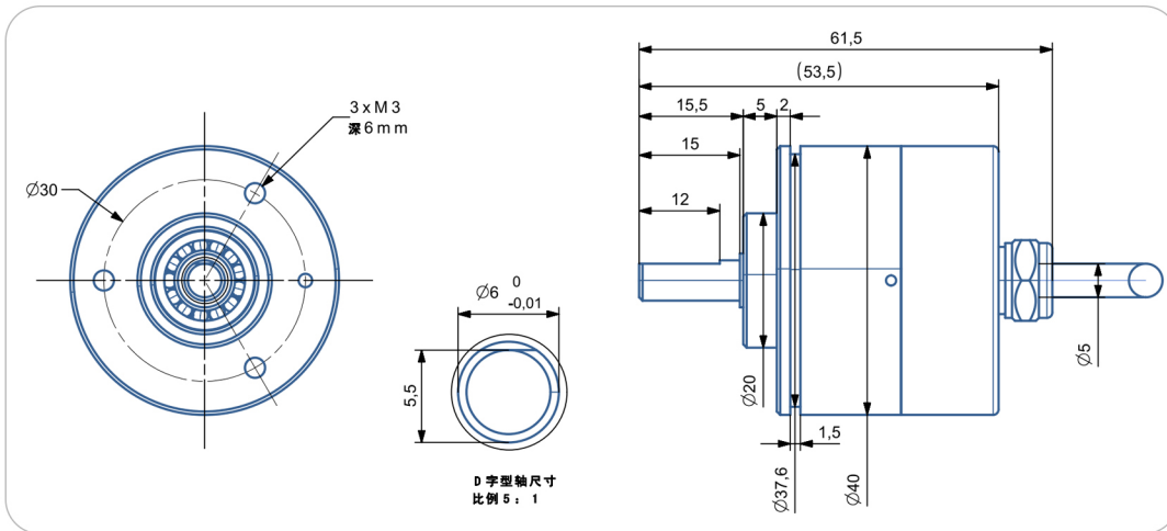
尺寸型号图6：输出轴6mm轴(尾出) IP68/防爆
