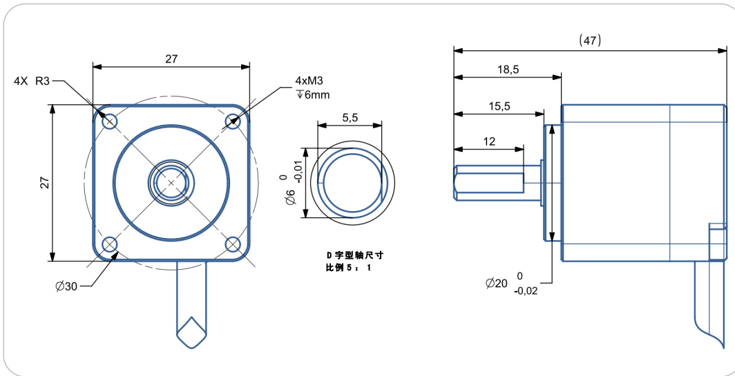
尺寸型号图8：输出轴6mm轴 IP68/防爆 (此形状编码器多圈圈数为：16/24/32/50/100/200/600圈)
