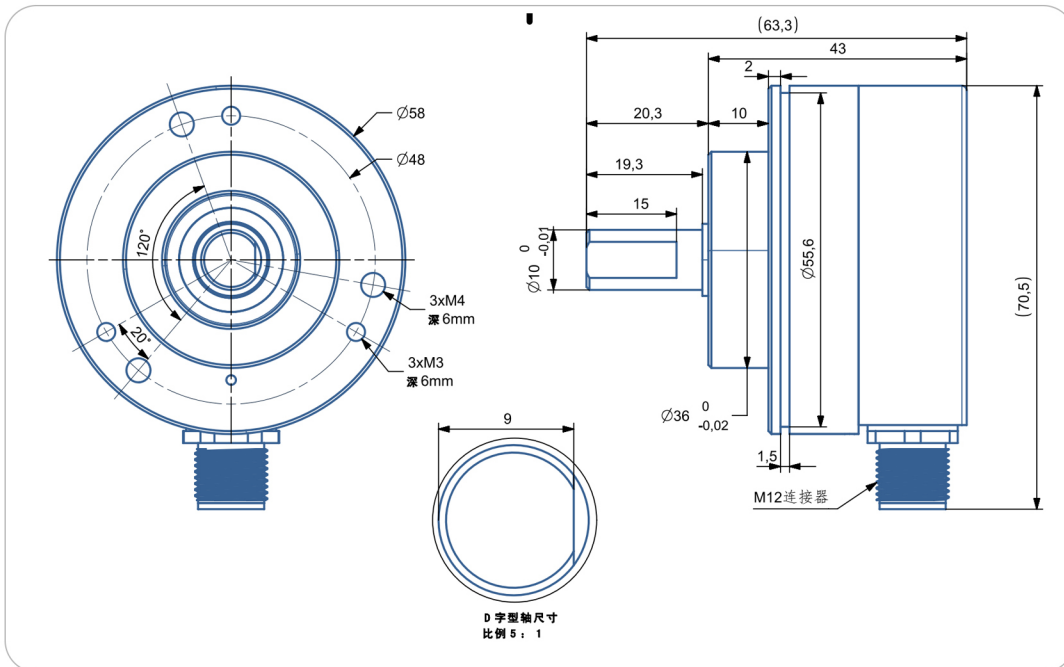
尺寸型号图9：输出轴10mm轴 P68/防爆
