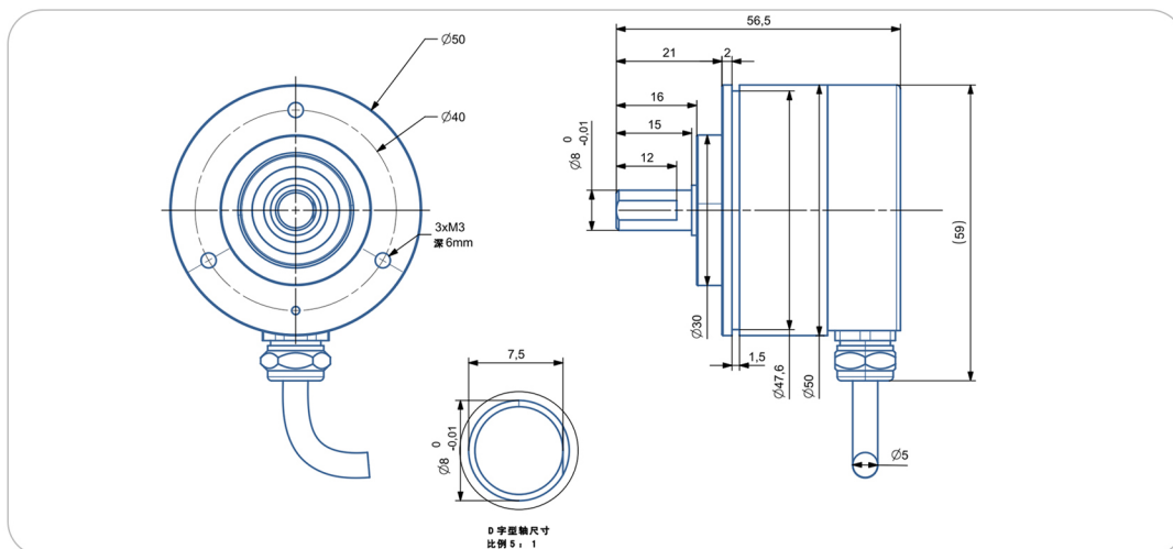
尺寸型号图7：输出轴8mm IP68/防爆
