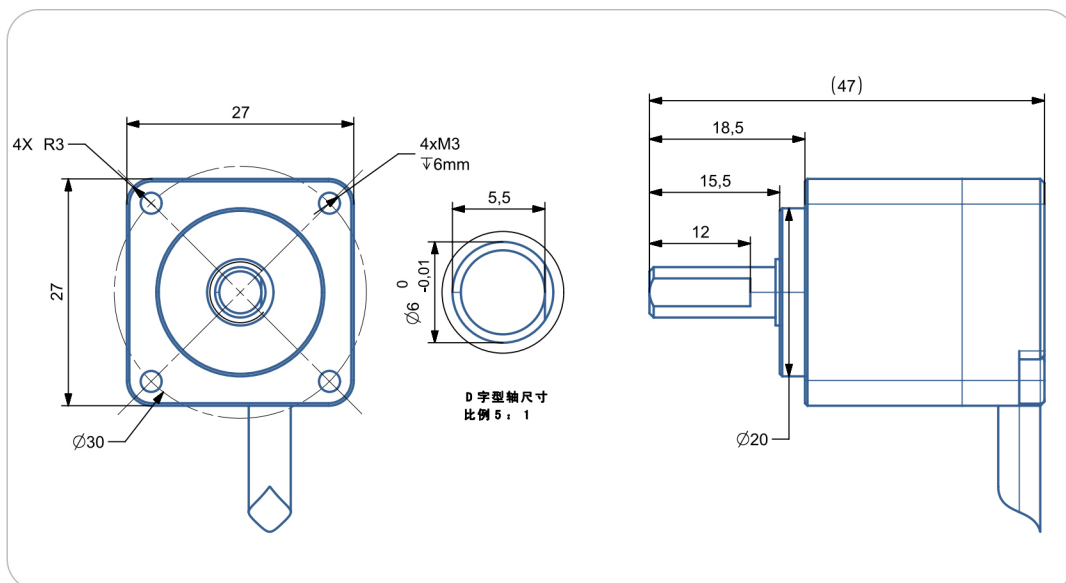
尺寸型号图8：输出轴6mm IP68/防爆 (此形状编码器多圈圈数为：16/24/32/50/100/200/600圈)
