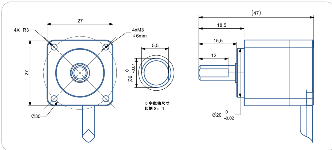
尺寸型号图11: 输出轴6mm轴 IP68/防爆
