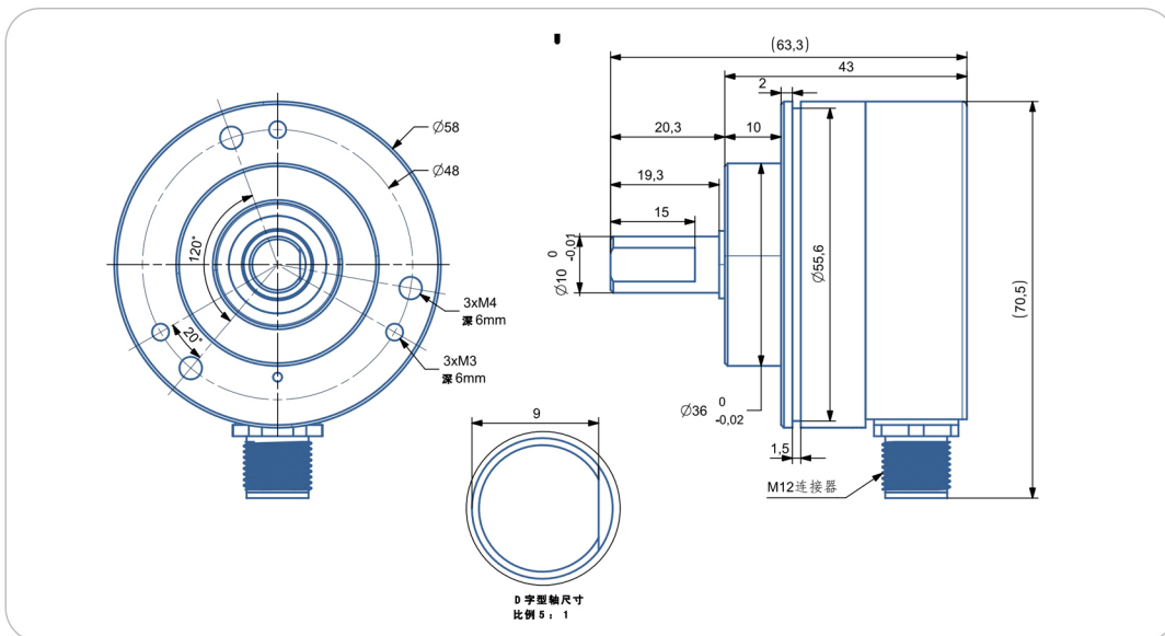
尺寸型号图12: 输出轴10mm IP54/IP68/防爆
