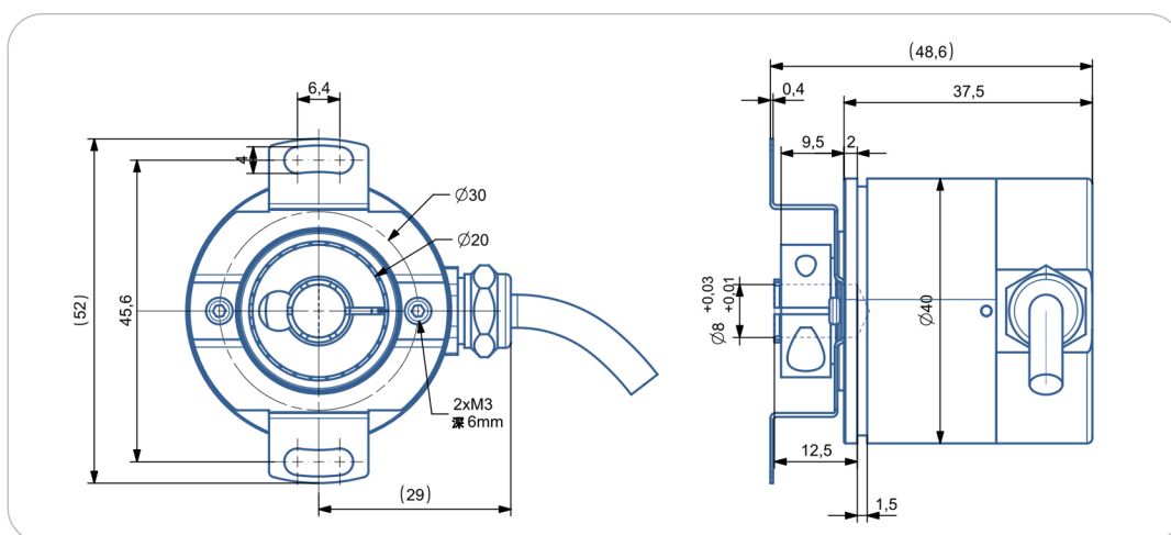
尺寸型号图9：输出轴8mm抱 IP68/防爆
