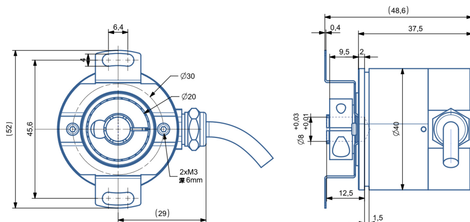
尺寸型号图9：输出轴8mm抱 IP68/防爆
