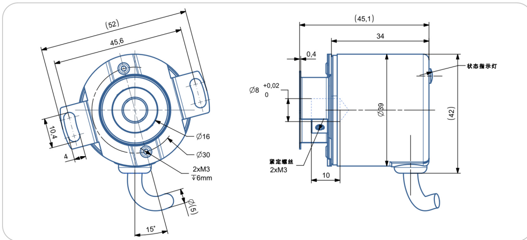
尺寸型号图3：输出轴8mm IP54
