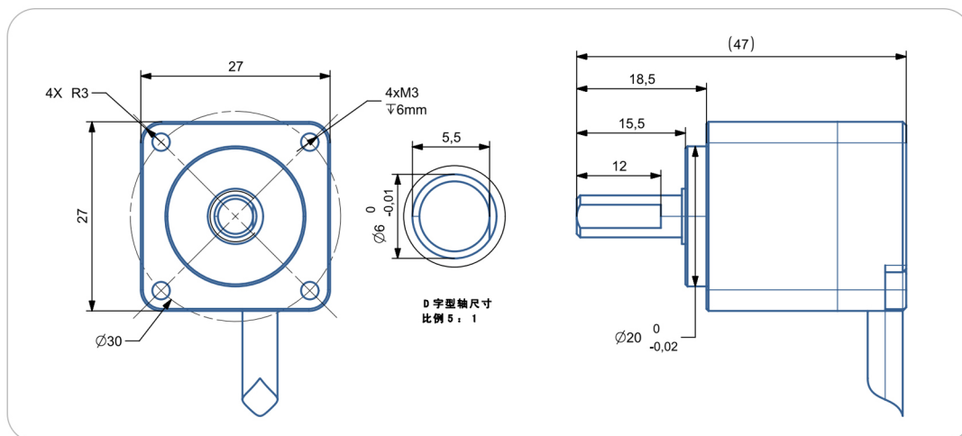
尺寸型号图11: 输出轴6mm IP68/防爆
