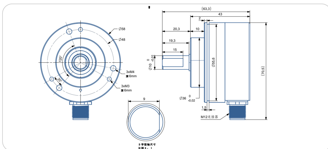
尺寸型号图12: 输出轴10mm轴 IP54/IP68/防爆
