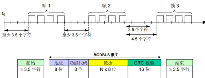
图 2-4 RTU 报文帧
