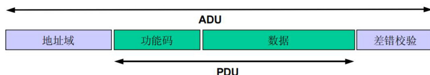
图 2-1 通用 MODBUS 帧
