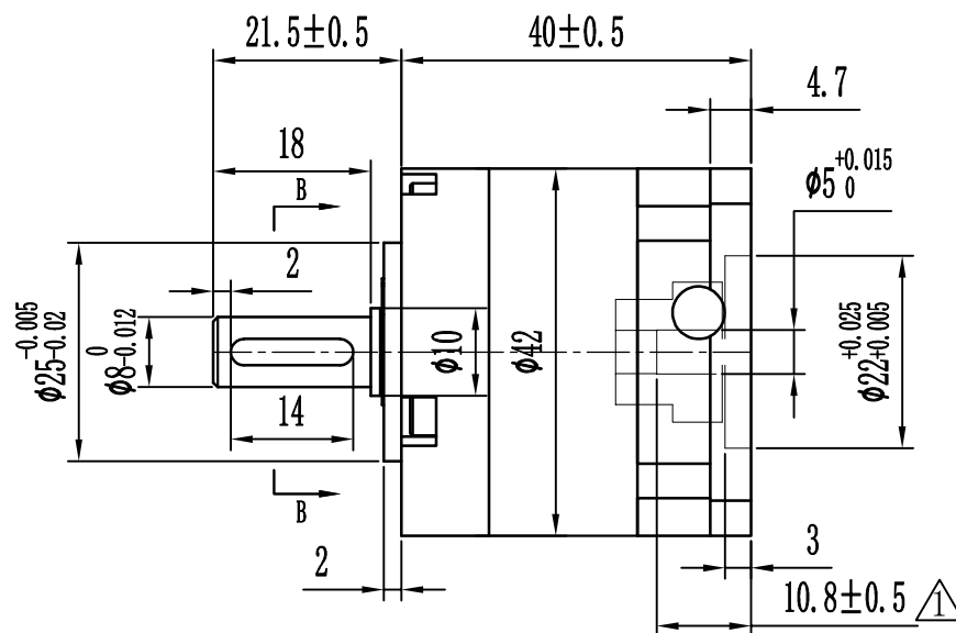
电机配合尺寸示意图
