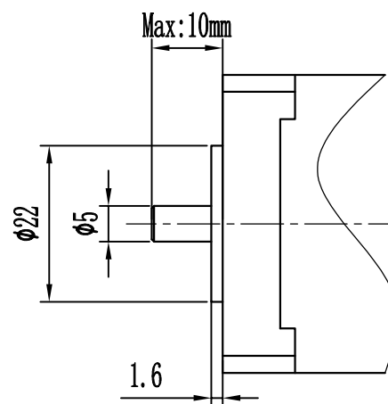
电机配合尺寸示意图
