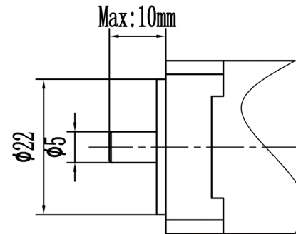
电机配合尺寸示意图 Motor size
